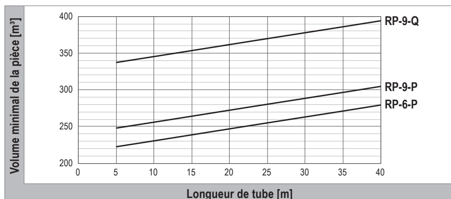
Image 3: Volume minimal de la pièce en fonction du volume de remplissage total de fluide frigorigène selon EN 378
