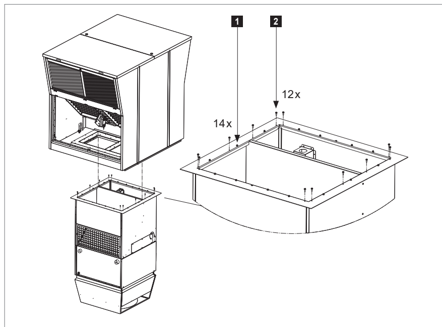
Image 32: Mise en place et montage de l'appareil de toiture
