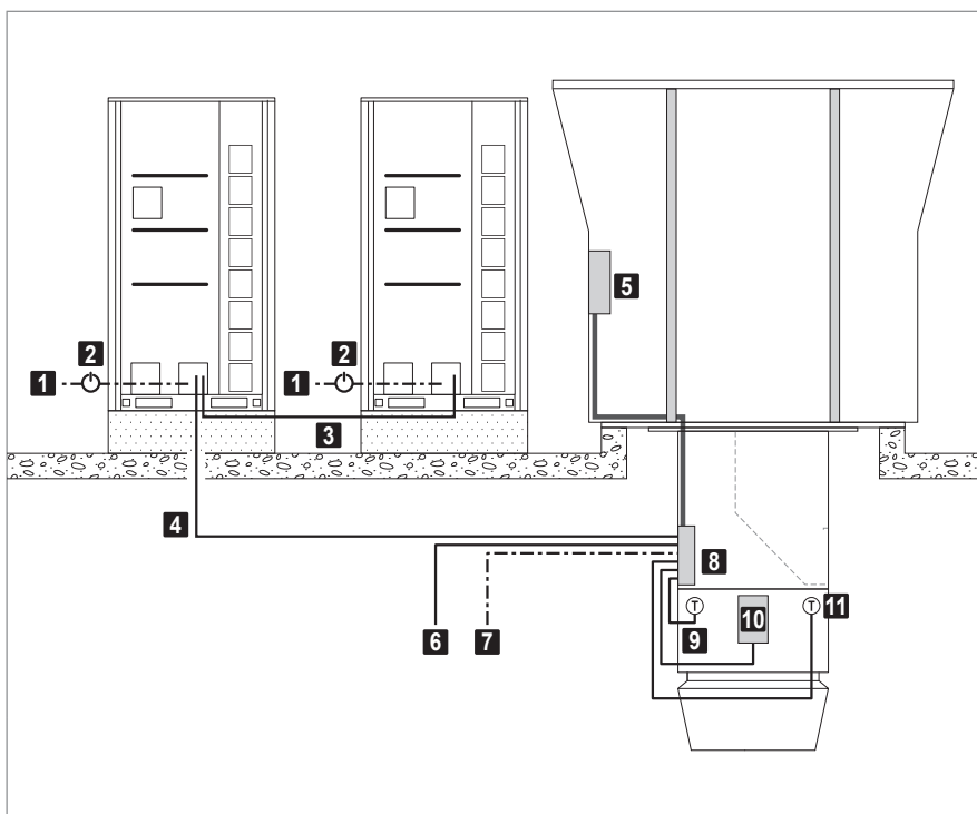
Image 55: Raccordement électrique du système de pompe à chaleur pour pompe à chaleur Q
