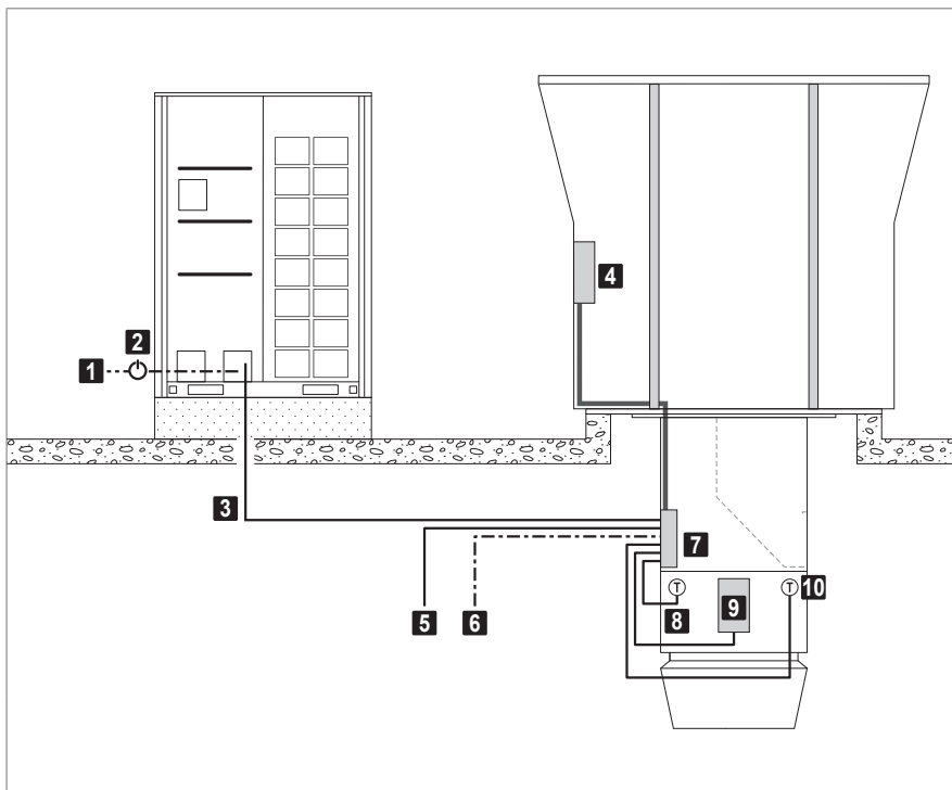
Image 54: Raccordement électrique du système de pompe à chaleur pour pompe à chaleur P
