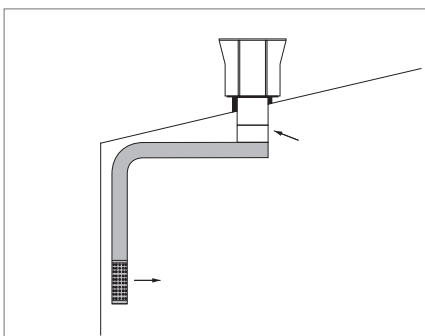
Image 10: Raccordement au système de diffusion externe
