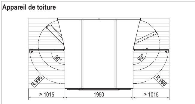
Image 13: Espace nécessaire pour la maintenance sur la toiture (dimensions en mm)
