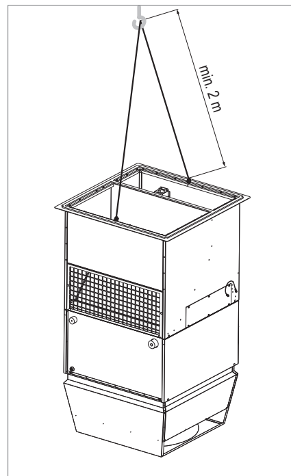
Image 28: Longueur minimale des câbles de levage
