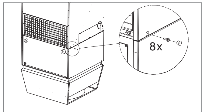
Image 22: Vissage de l'élément sous-toiture avec des vis M6 x 20 et des capuchons (8x par composant)
