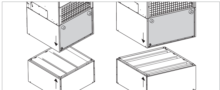
Image 24: Positionnement correcte de l'atténuateur sonore pour l'air pulsé: pour taille 6: coulisses absorbantes transversalement au côté du raccord de fluide frigorigène pour taille 9: coulisses absorbantes parallèlement au côté du raccord de fluide frigorigène
