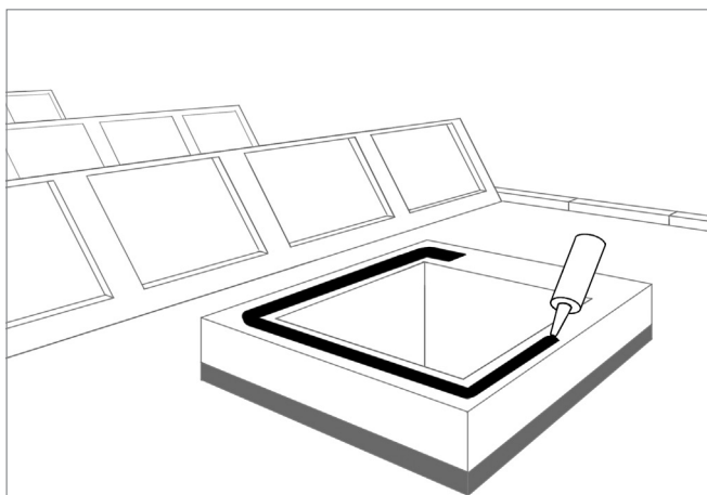
Image 29: Application de produit d'étanchéité sur le socle de toiture
