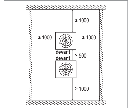
Image 16: Distances minimales pour la pompe à chaleur Q (dimensions en mm)
