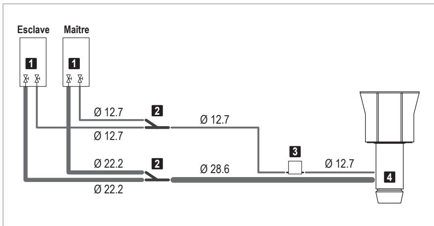
Image 44: Conduites frigorifiques pour pompe à chaleur Q (diamètre de conduite en mm)
