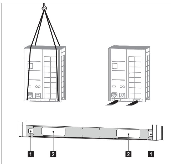
Image 12: Levage de la pompe à chaleur
