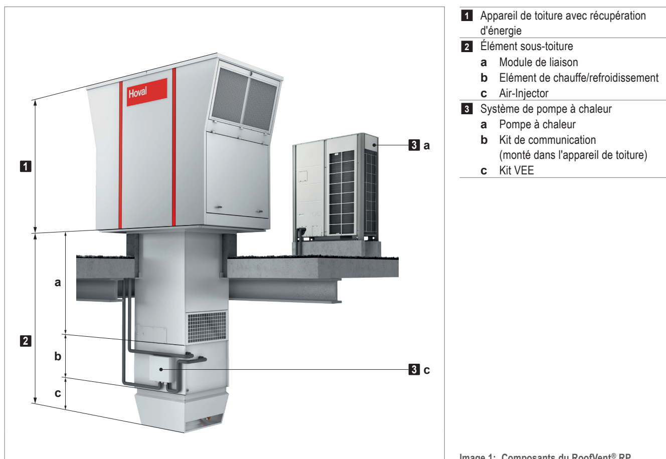
Image 1: Composants du RoofVent® RP
