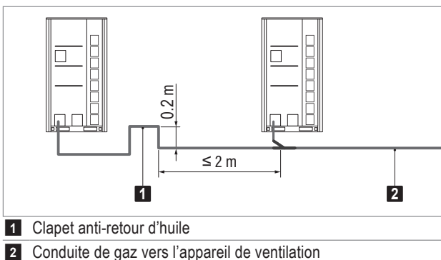
Image 47: Clapet anti-retour d'huile
