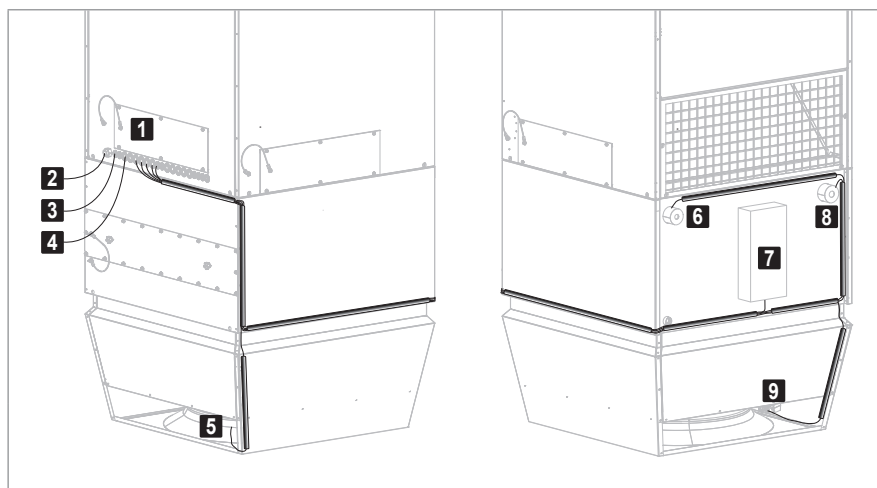
Image 56: Cheminement des câbles au niveau de l'élément sous-toiture
