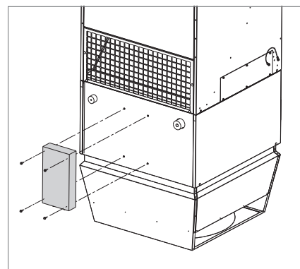
Image 35: Montage du kit VEE
