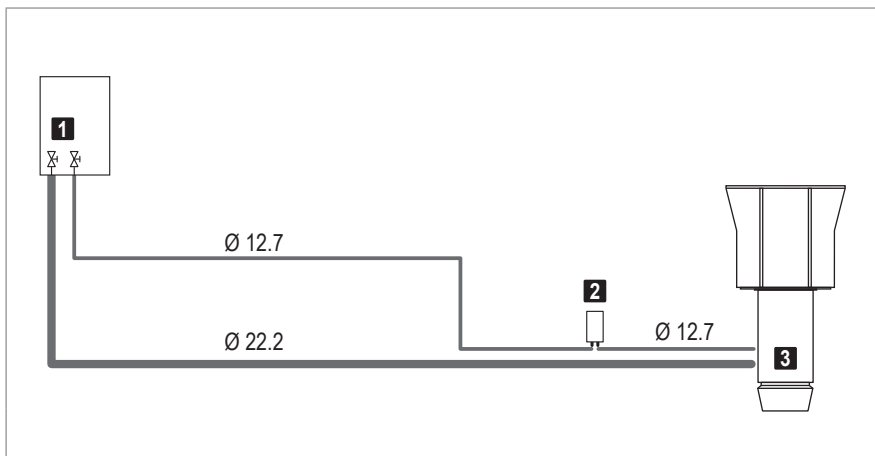
Image 43: Conduites frigorifiques pour pompe à chaleur P (diamètre de conduite en mm)
