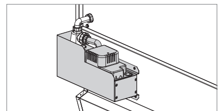
Fig. B16: Montage sur l'appareil
