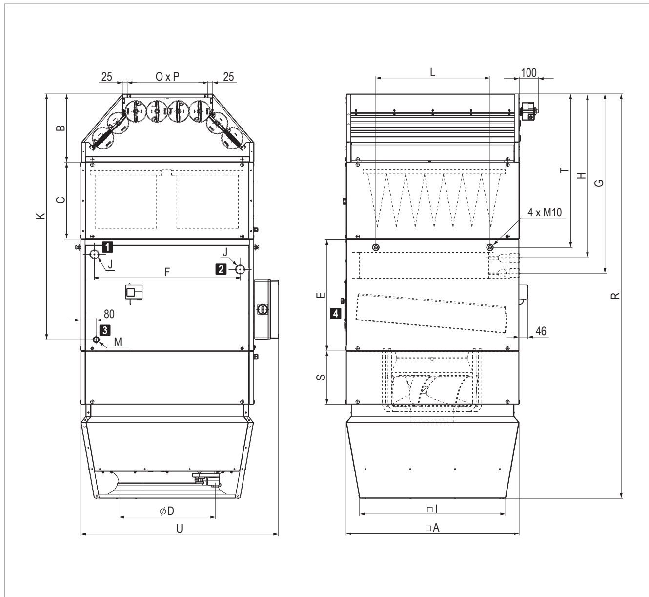
Fig. B7: Dimensions du TopVent® MC
