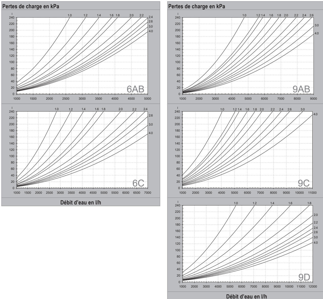
Fig. B13: Valeurs de réglage des vannes de régulation
