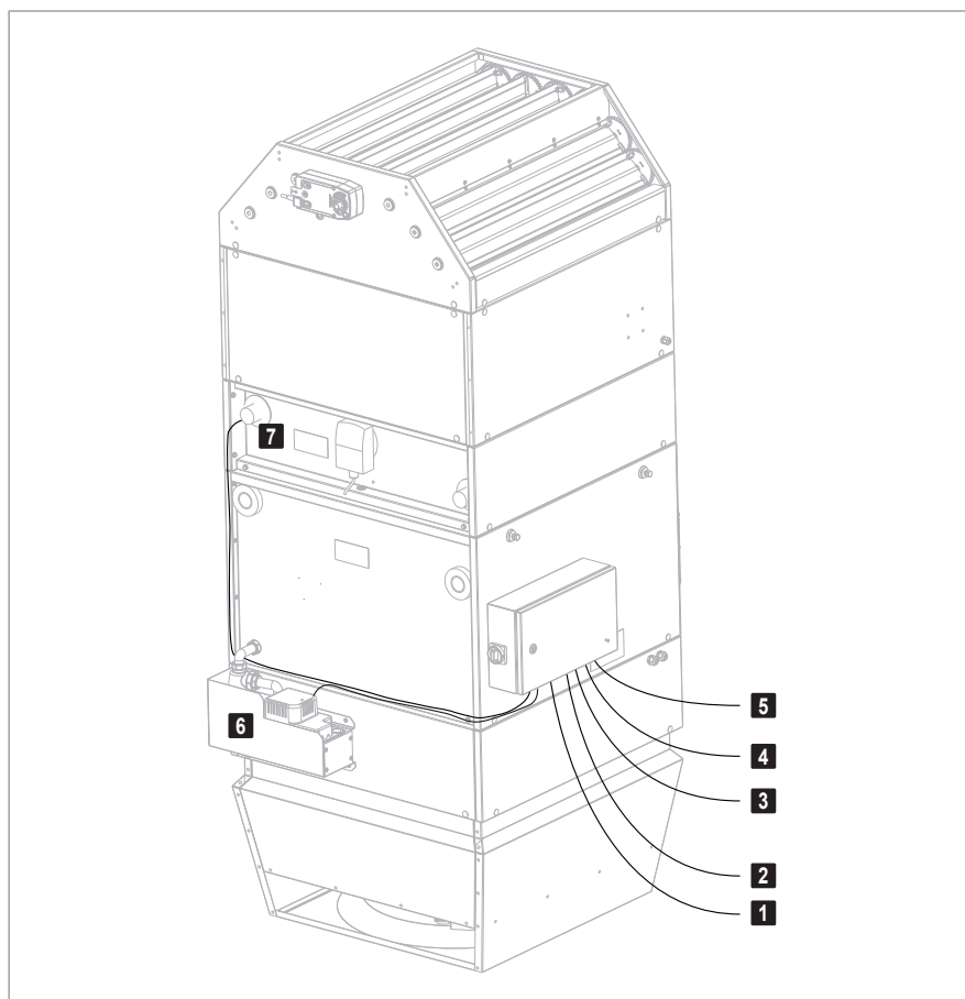
Fig. B19: Raccordement électrique sur site des appareils d'introduction d'air TopVent®
