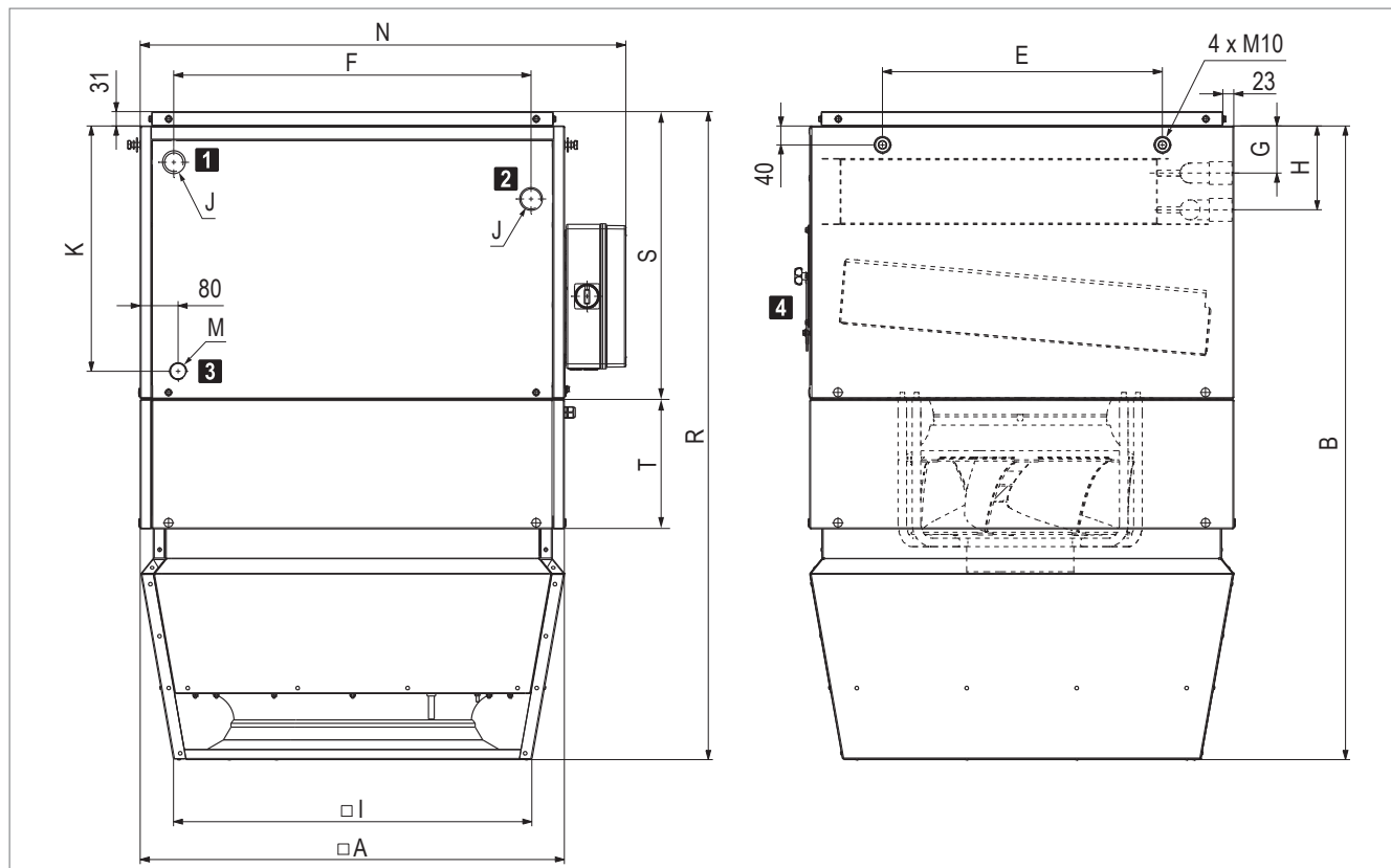
Fig. B4: Dimensions du TopVent® TC
