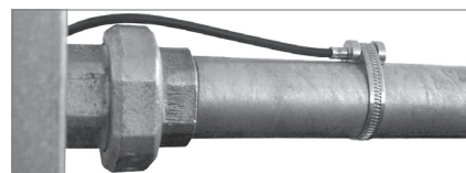
Fig. B14: Sonde de température de retour
