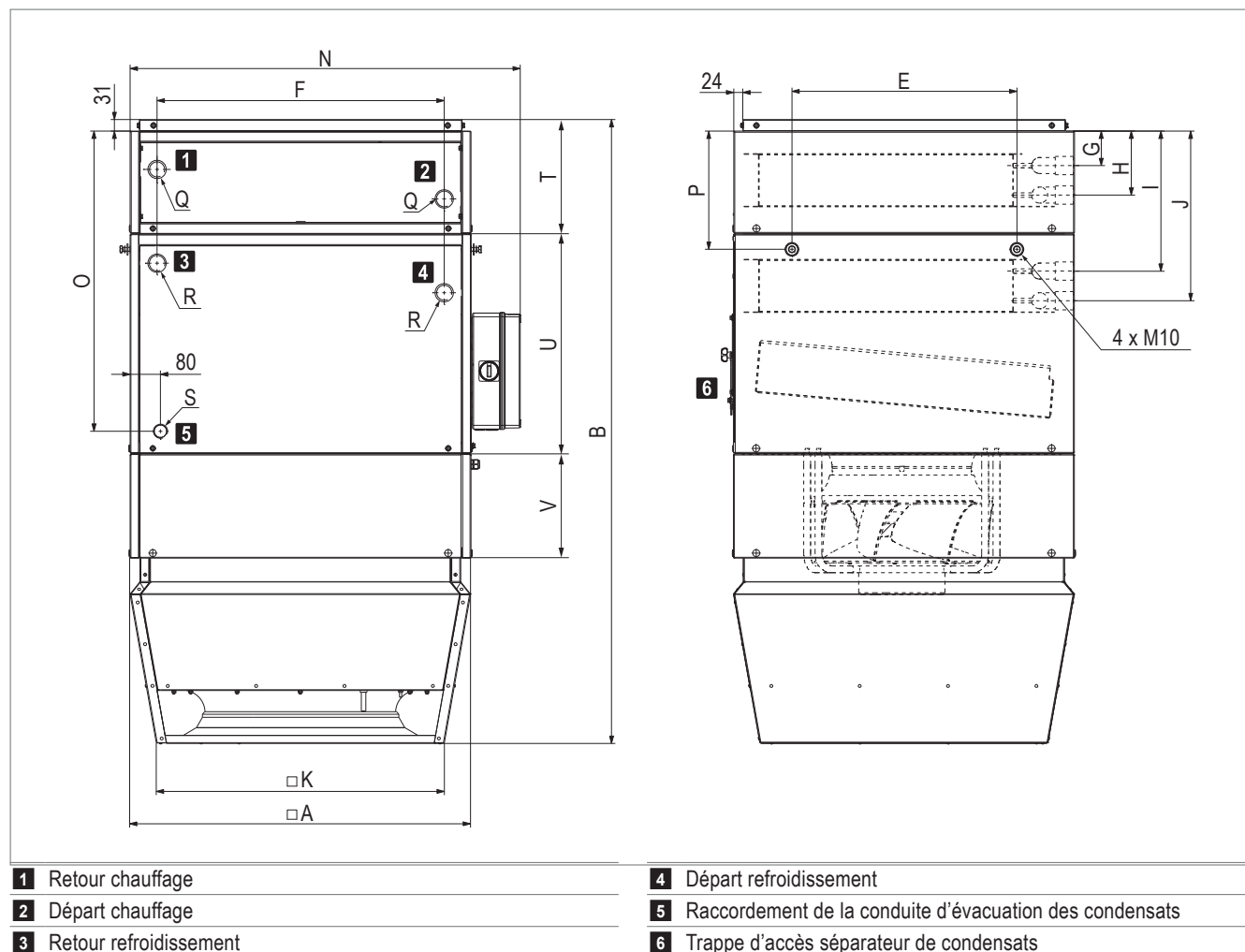
Fig. B5: Dimensions du TopVent® THC
