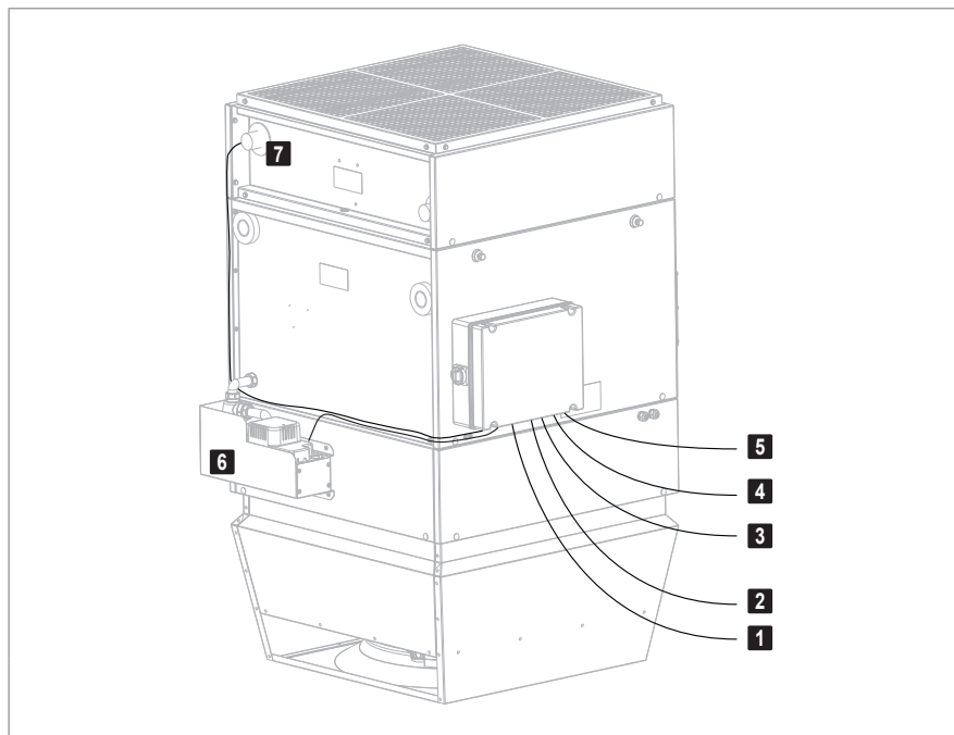
Fig. B18: Raccordement électrique sur site des appareils de recyclage d'air TopVent®
