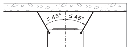
Fig. B12: Suspension inclinée sur les côtés
