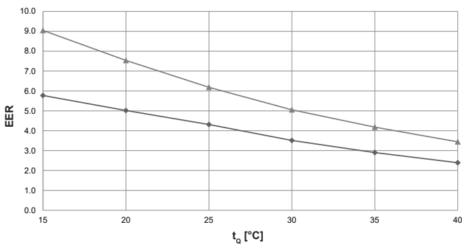
Coefficient d'efficacité énergétique – t_{VL} 18\text{ °C}
