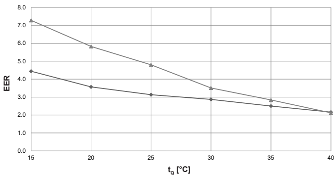
Coefficient d'efficacité énergétique – t_{VL} 12\text{ °C}
