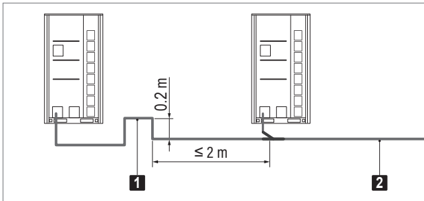
Image E15: Clapet anti-retour d'huile
