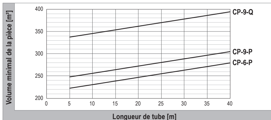
Image B4: Volume minimal de la pièce en fonction du volume de remplissage total de fluide frigorigène selon EN 378
