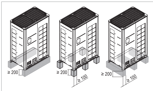
Image E7: Socle pour la pompe à chaleur
