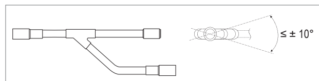
Image E14: Installation du kit de branchement
