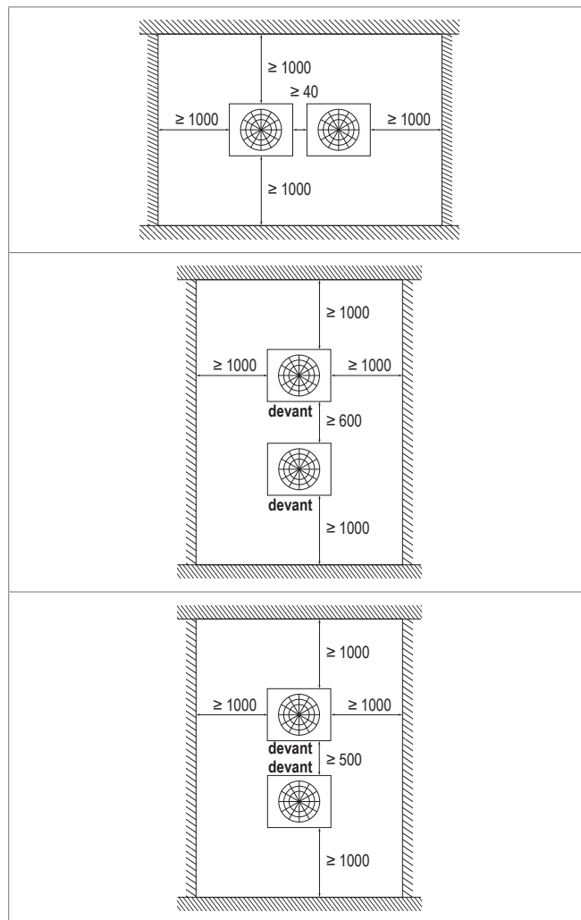
Image E6: Distances minimales pour la pompe à chaleur Q (dimensions en mm)
