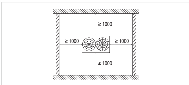
Image E5: Distances minimales pour la pompe à chaleur P (dimensions en mm)
