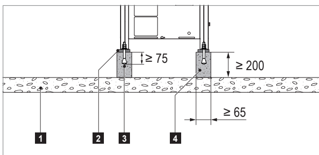
Image E7: Socle pour la pompe à chaleur
