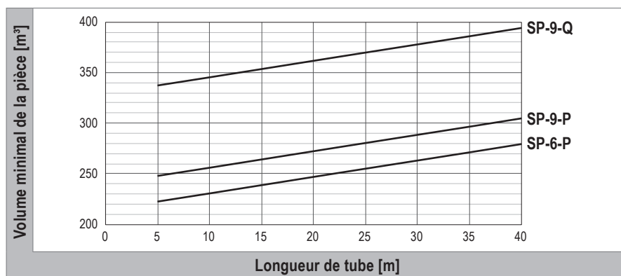
Image C3: Volume minimal de la pièce en fonction du volume de remplissage total de fluide frigorigène selon EN 378
