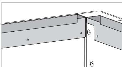
Image D4: Rails de fixation pour la membrane
