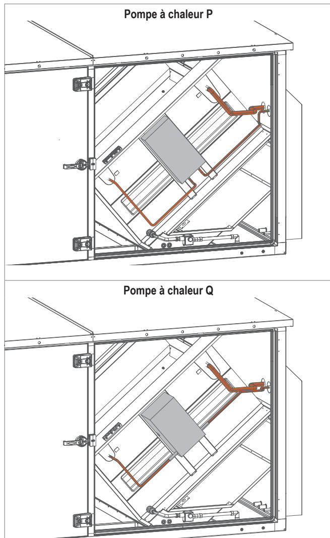
Image E12: Installation des conduites frigorifiques dans l'appareil de toiture
