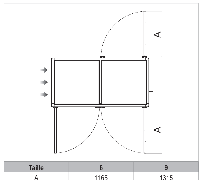
Image E3: Espace nécessaire pour l'ouverture des portes de révision (dimensions en mm)
