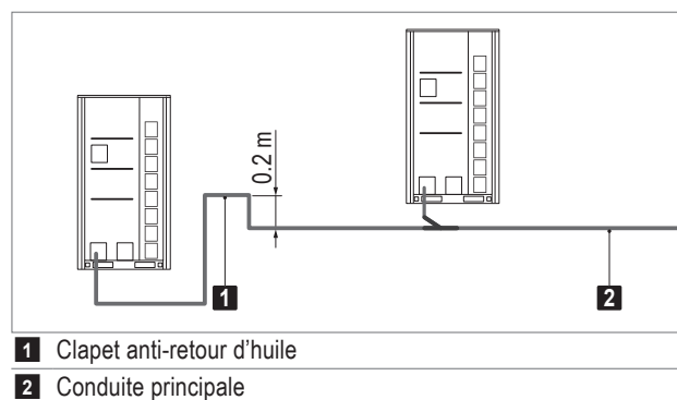
Image E13: Clapet anti-retour d'huile
