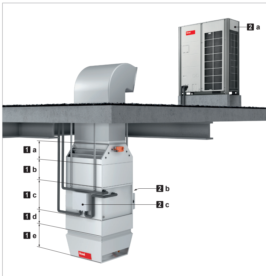
Fig. D1: Composants du TopVent® MP
