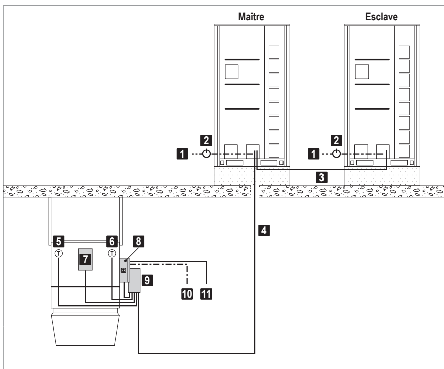
Fig. F15: Raccordement électrique du système de pompe à chaleur pour pompe à chaleur Q
