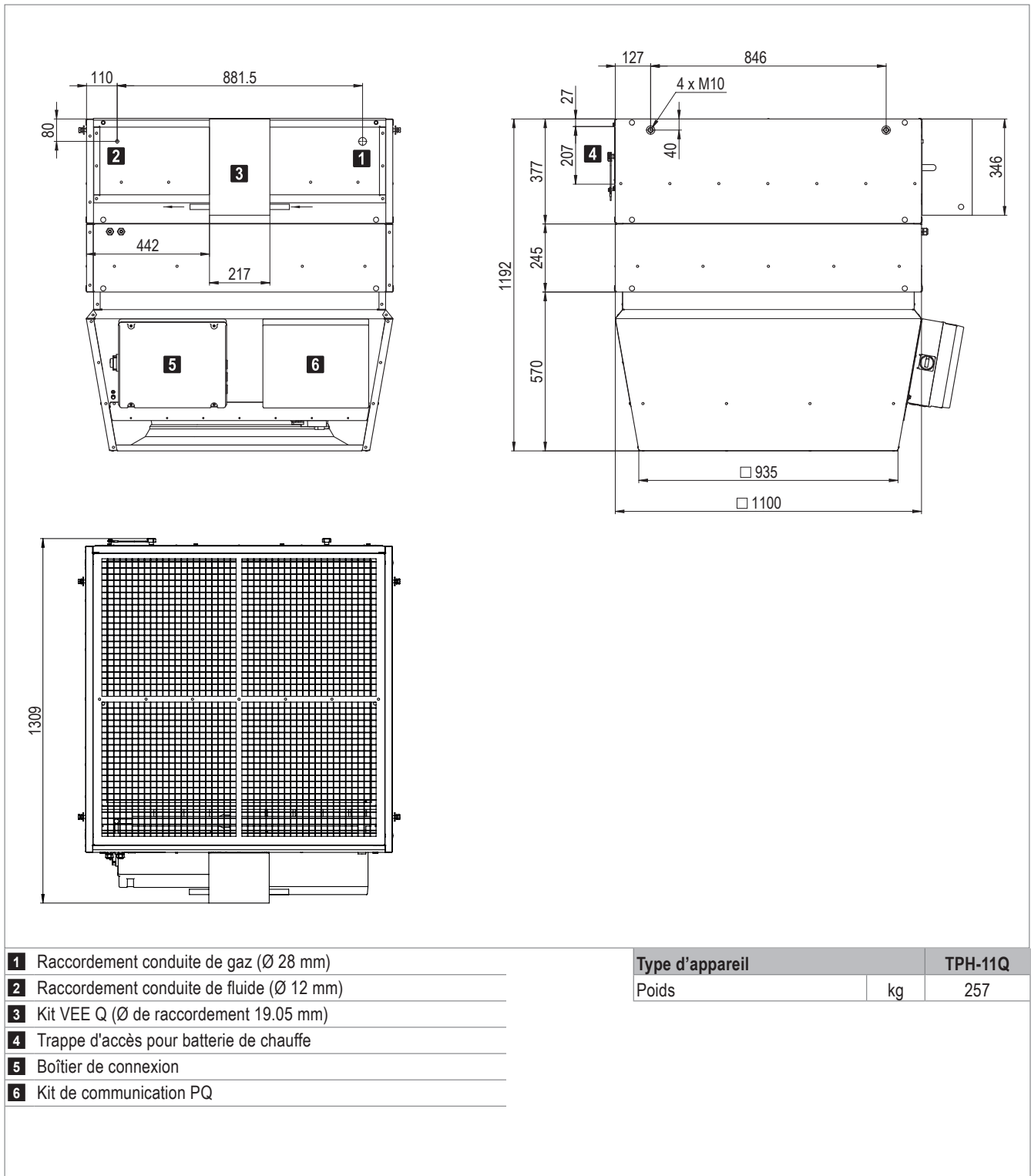
Fig. C8: Dimensions et poids du TopVent® TPH-11Q
