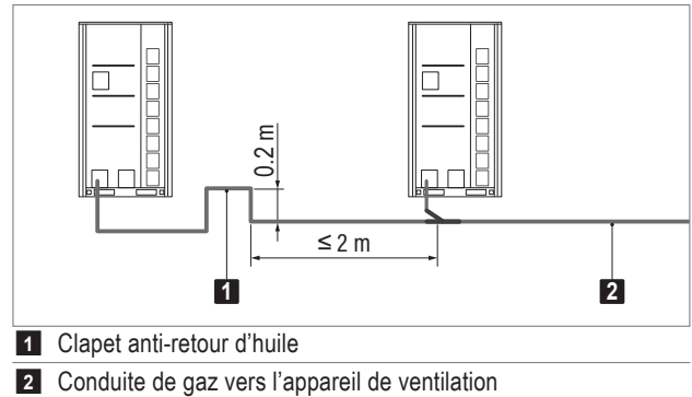
Fig. F11: Clapet anti-retour d'huile
