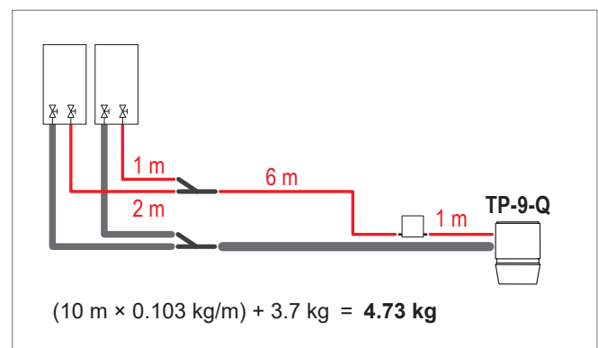
Fig. F12: Exemple de calcul
