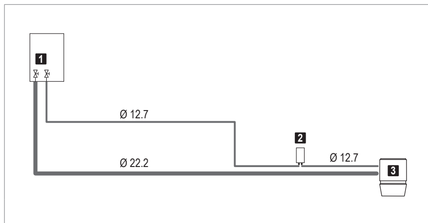
Fig. F7: Conduites frigorifiques pour pompe à chaleur P (diamètre de conduite en mm)
