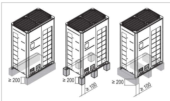
Fig. F5: Socle pour la pompe à chaleur
