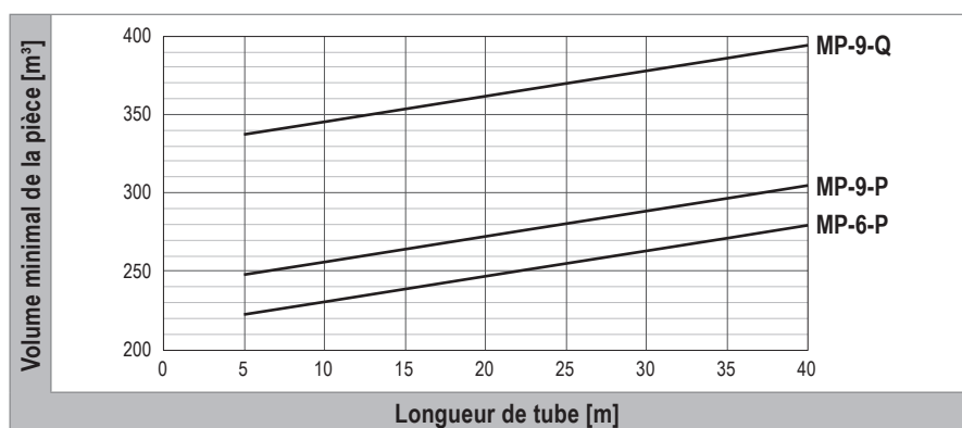
Fig. D5: Volume minimal de la pièce en fonction du volume de remplissage total de fluide frigorigène selon EN 378
