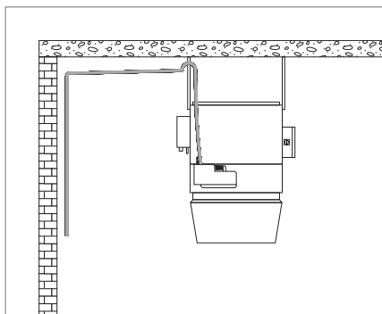
Fig. F13: Conduite d'évacuation des condensats
