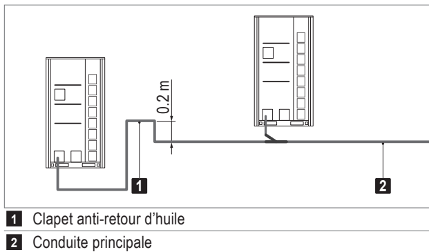
Fig. F9: Clapet anti-retour d'huile
