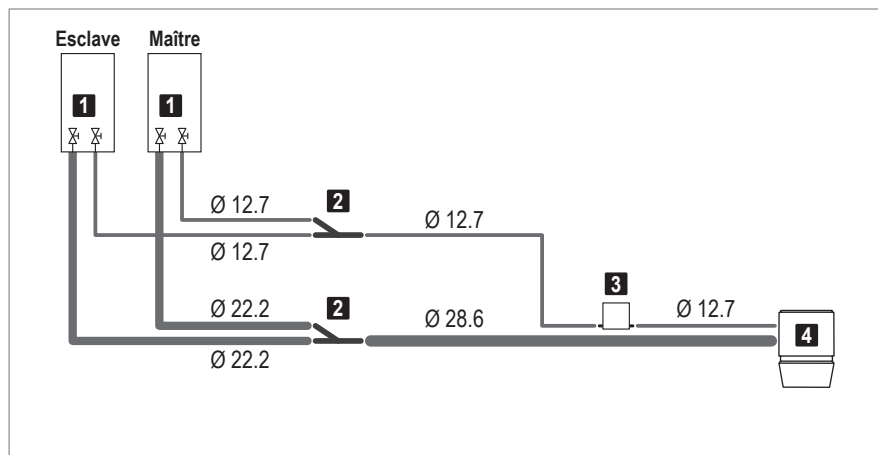
Fig. F8: Conduites frigorifiques pour pompe à chaleur Q (diamètre de conduite en mm)
