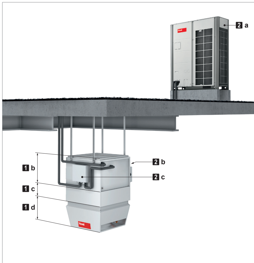
Fig. B1: Composants du TopVent® TP
