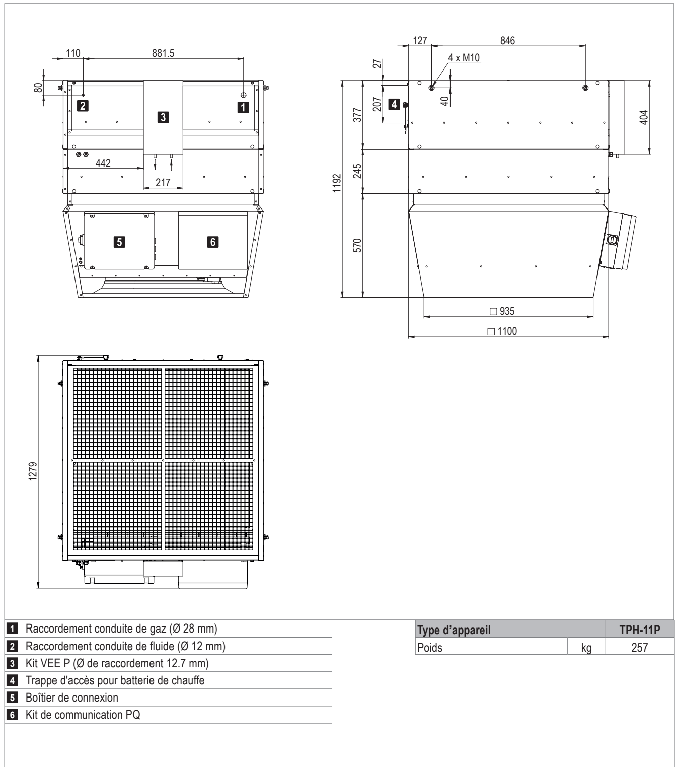
Fig. C6: Dimensions et poids du TopVent® TPH-11P
