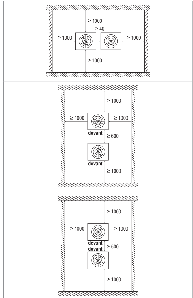
Fig. F4: Distances minimales pour la pompe à chaleur Q (dimensions en mm)
