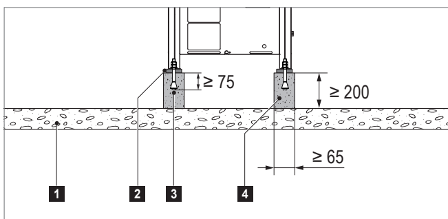
Fig. F5: Socle pour la pompe à chaleur
