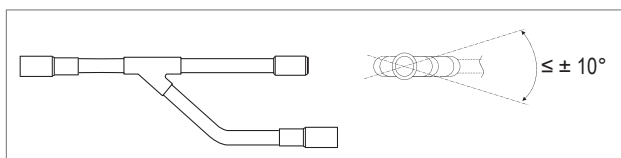
Fig. F10: Installation du kit de branchement
