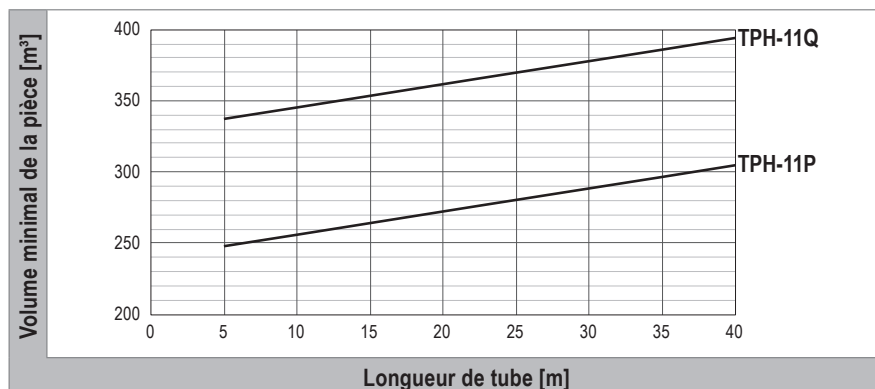
Fig. C5: Volume minimal de la pièce en fonction du volume de remplissage total de fluide frigorigène selon EN 378
