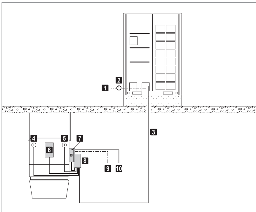
Fig. F14: Raccordement électrique du système de pompe à chaleur pour pompe à chaleur P
