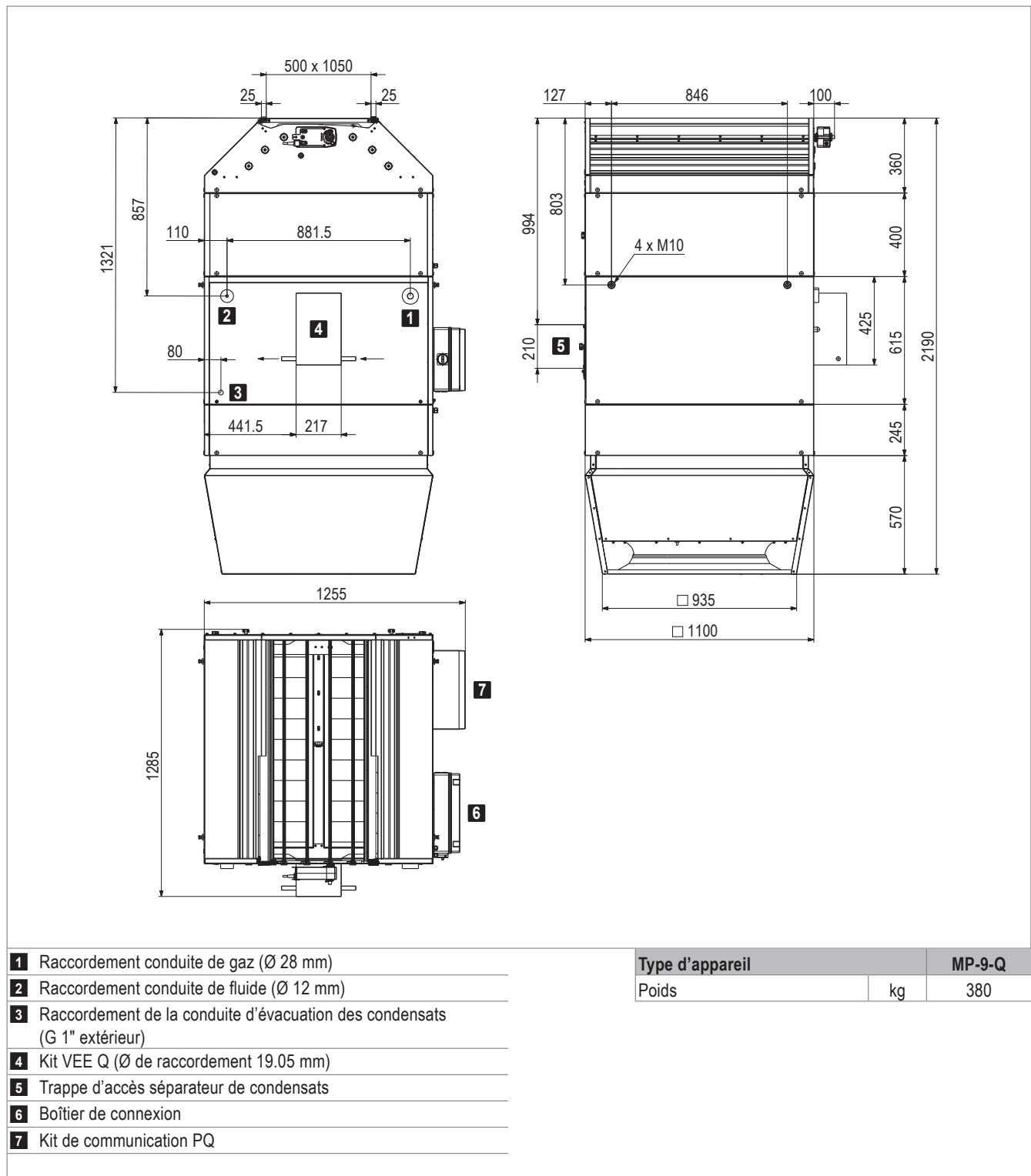
Fig. D9: Dimensions et poids du TopVent® MP-9-Q
