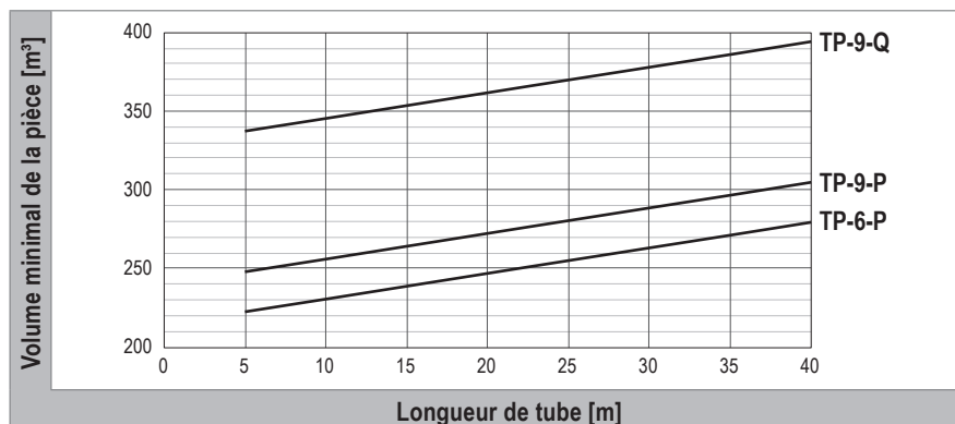
Fig. B5: Volume minimal de la pièce en fonction du volume de remplissage total de fluide frigorigène selon EN 378
